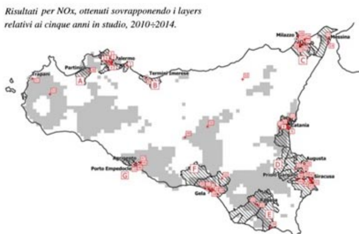
Figura 2: Indice FEAI valutato per NO x (in grigio affinità Alta; in bianco bassa)
