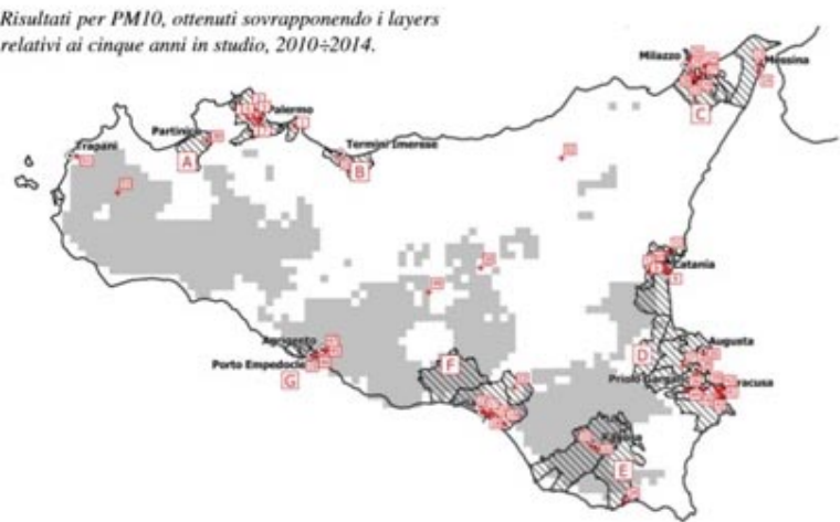
Figura 3: Indice FEAI valutato per PM10 (in grigio affinità Alta; in bianco bassa)
