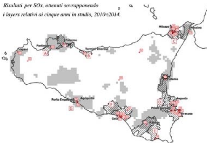
Figura 1: Indice FEAI valutato per SO x (in grigio affinità Alta; in bianco bassa)
